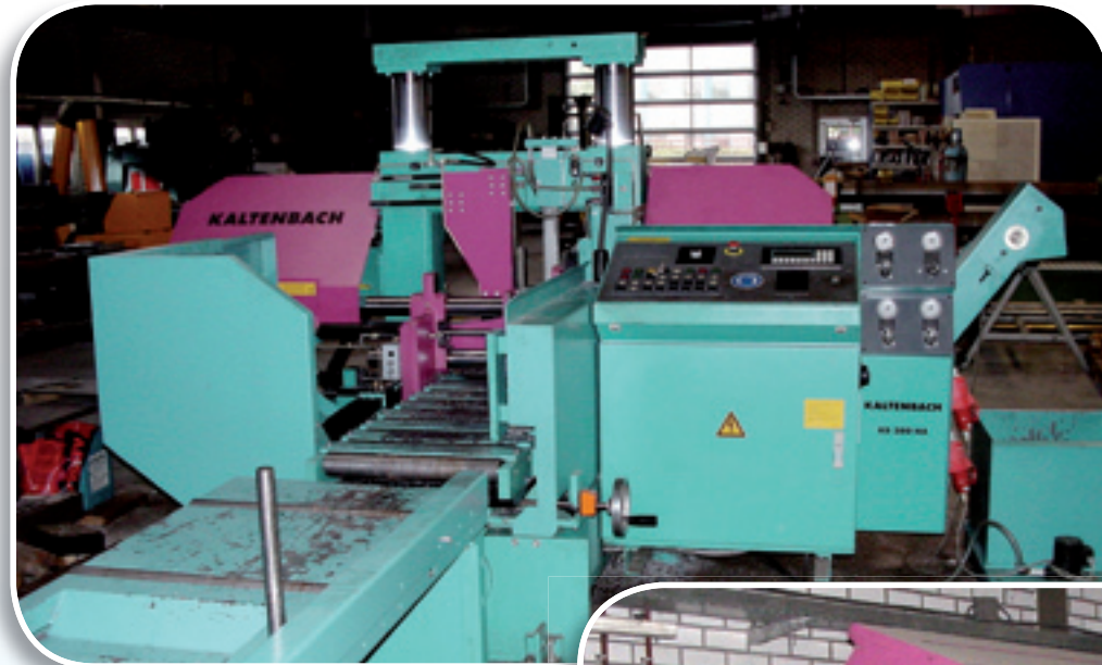
Kaltenbach type KB380NA bandzaag machine bewerkingscapaciteit 380 mm Auto feeder
