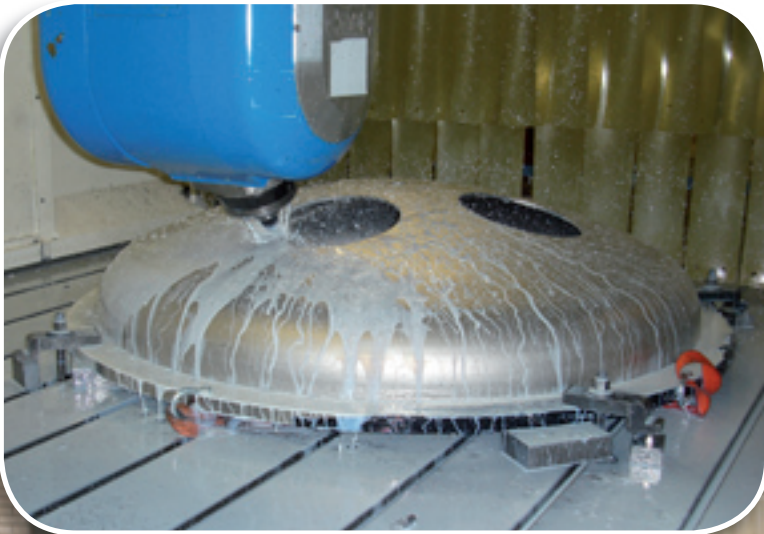
Edel Portaal bewerkingsunit type Cyport CP 3020 40 gereedschappen wisselaar bedafmetingen 5000 x 2310 mm bewerkingscapaciteit 3000 x 2000 x 960 mm.
