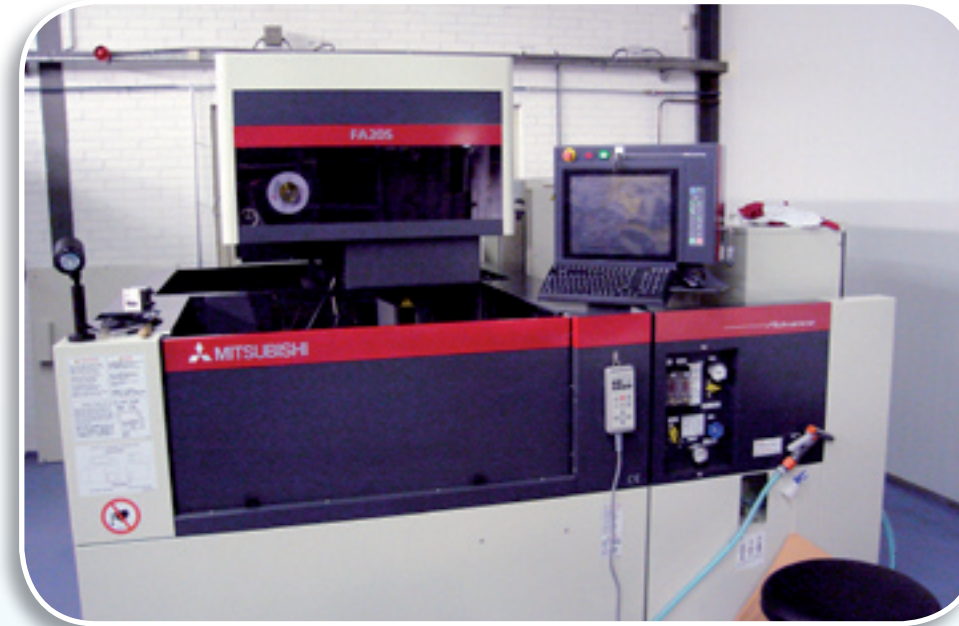
Mitsubishi Electric type FA 20 S Advance Draaderodeer machine bewerkingscapaciteit 500 x 350 x 300 mm
